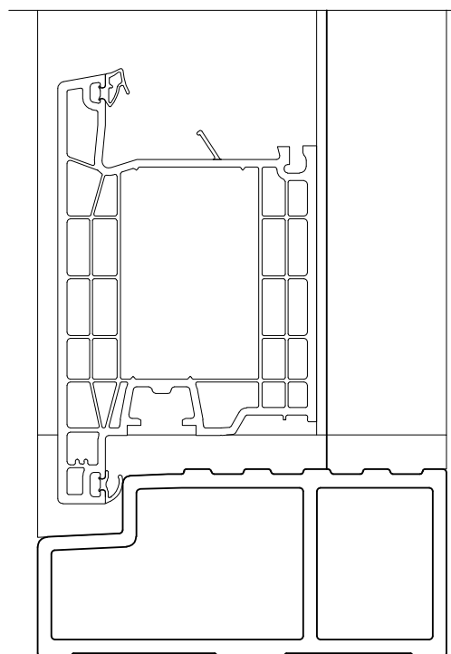
Buitendraaiend verdiept
