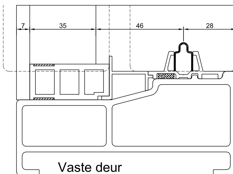
Schuivende deur hoge looprail Detail A
