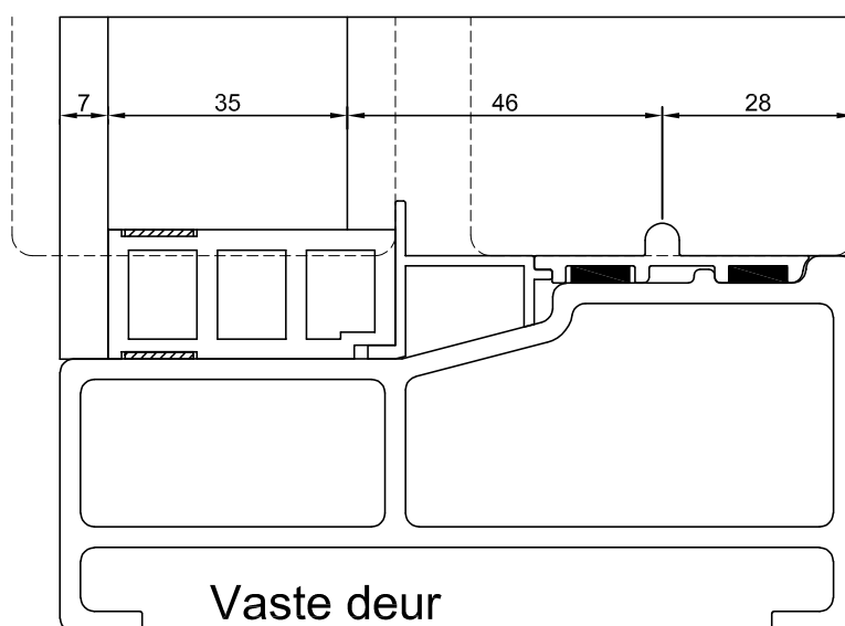
Schuivende deur lage looprail Detail B
