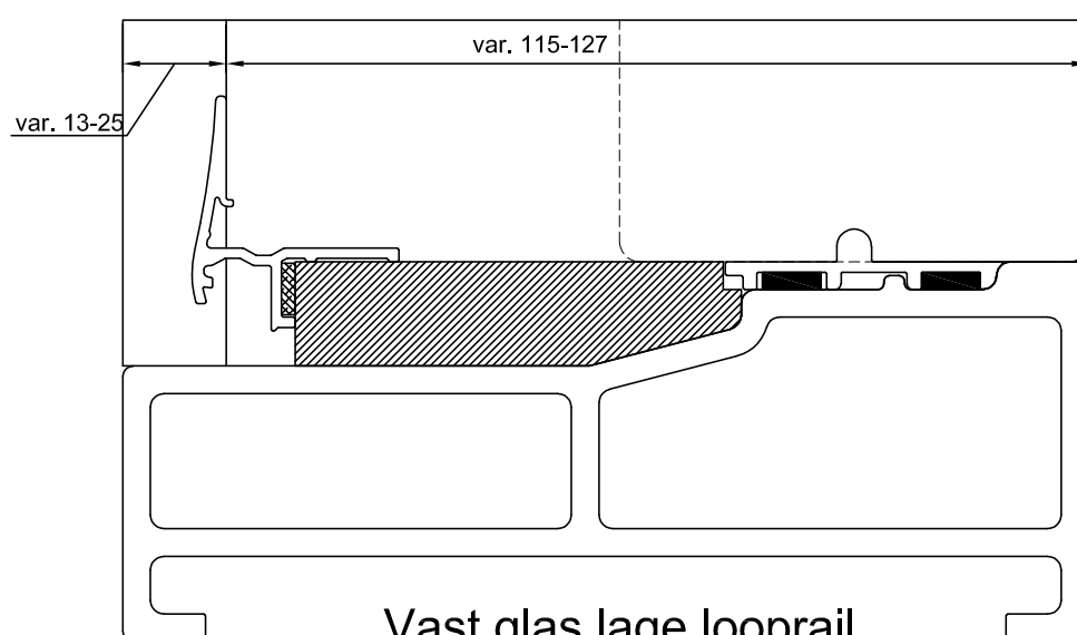
Vast glas hoge looprail zonder kozijn-tussenstijl Detail F
