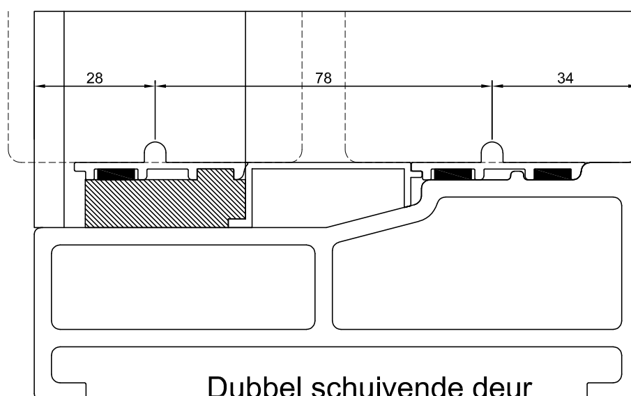
Dubbel schuivende deur met lage looprail Detail P
