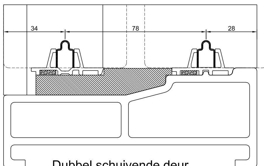
Dubbel schuivende met deur hoge looprail Detail LL
