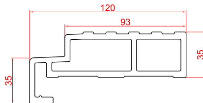
EEAL INHAAK VOOR ALUPLAST (BUITENDRAAIEND)
