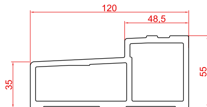
EEAL VOOR ALUPLAST (BINNENDRAAIEND)
