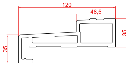
EEAL INHAAK VOOR ALUPLAST (BINNENDRAAIEND)
