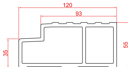
EEAL VOOR ALUPLAST (BUITENDRAAIEND)
