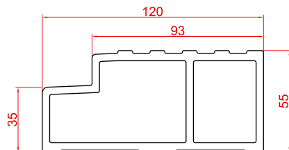
EEAL VOOR GEALAN (BUITENDRAAIEND)
