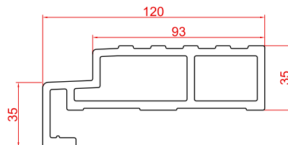
EEAL INHAAK VOOR GEALAN (BUITENDRAAIEND)
