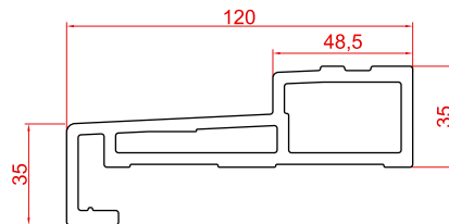
EEAL INHAAK VOOR GEALAN (BINNENDRAAIEND)
