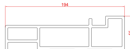
EEAS VOOR GEALAN (HEFSCHUIF OPLOSSING)
