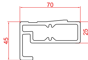
EEVD VOOR SCHÜCO CT-70 (VLAKPROFIEL OPLOSSING)
