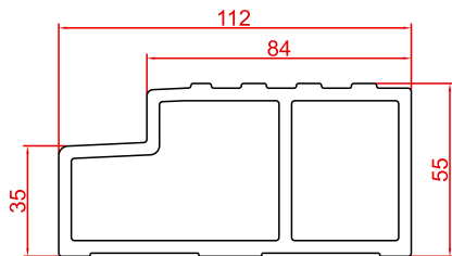
EEAL VOOR SCHÜCO ACCENT (BUITENDRAAIEND)
