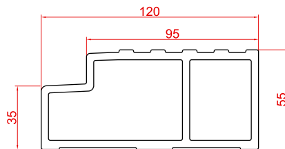
EEAL VOOR SCHÜCO LivIng (BUITENDRAAIEND)
