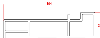
EEAS VOOR SCHÜCO (HEFSCHUIF OPLOSSING)
