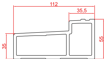
EEAL VOOR SCHÜCO ACCENT (BINNENDRAAIEND)
